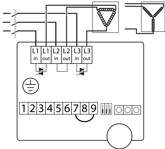
Abb. 1: Anschluss der Versorgungsspannung und Last
