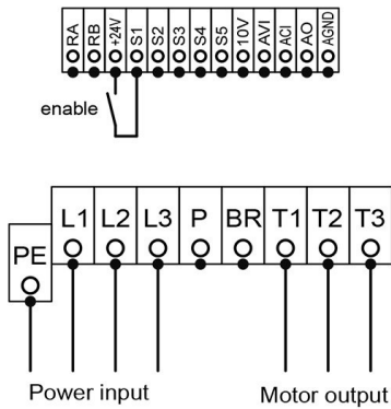
Wiring diagram:
