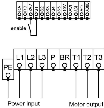
Wiring diagram:
