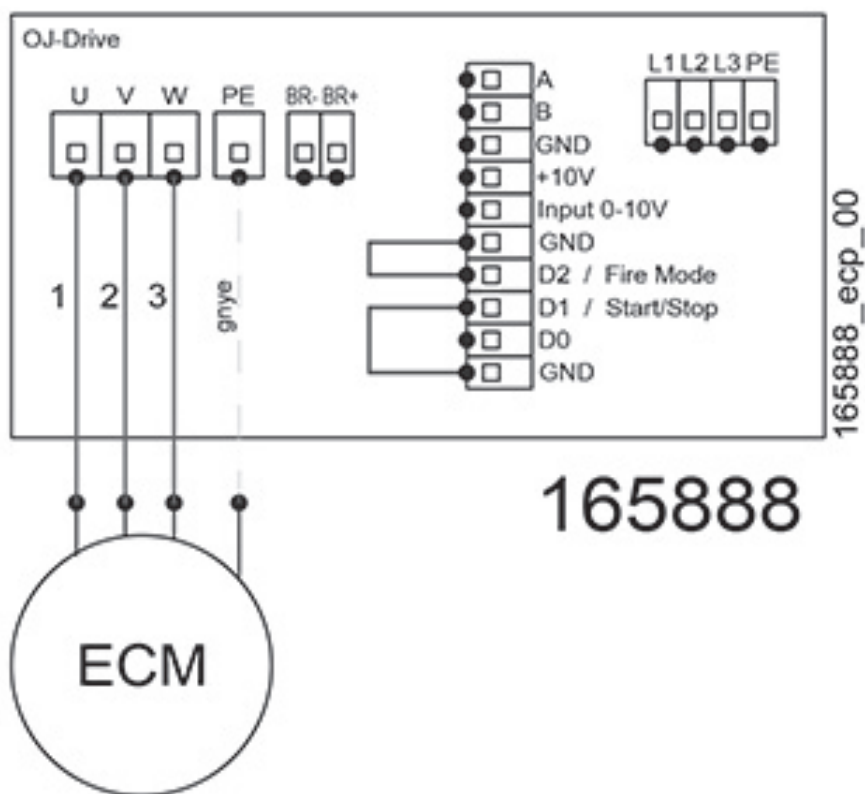
Anschluss 0-10V Signal
