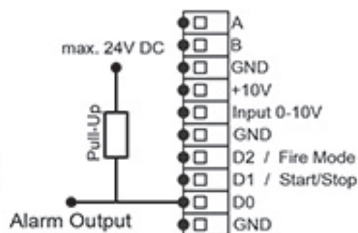
Anschluss Alarmausgang
