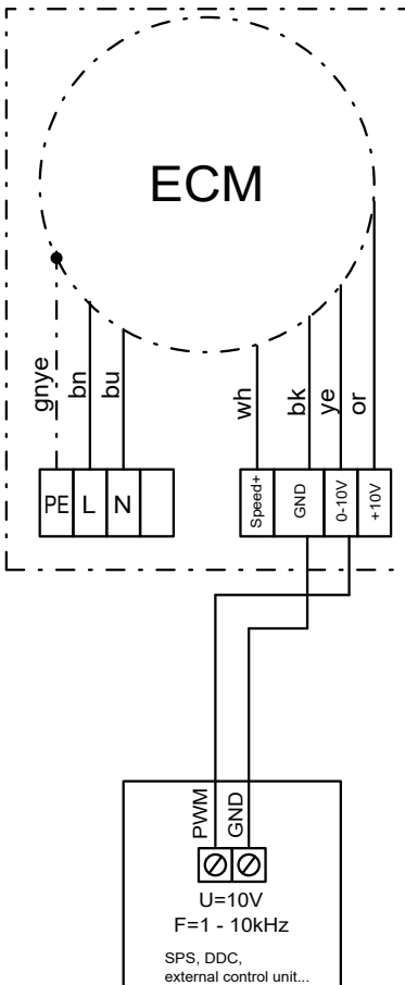
Aansluiting PWM-siganaal
