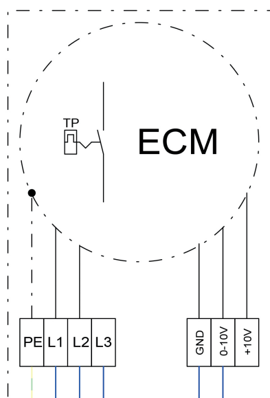
EC Motor 3~
