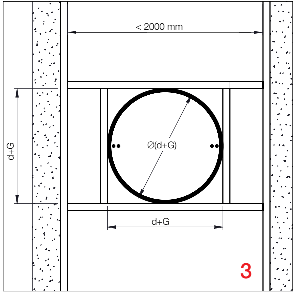
E-FDC-MF2 Installazione della serranda tagliafuoco in parete di vani (90 mm) senza borchie metalliche (larghezza massima della parete: 2000 mm)
