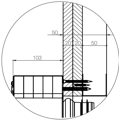
E-FDC25, E-FDC40 - sezione trasversale laterale
