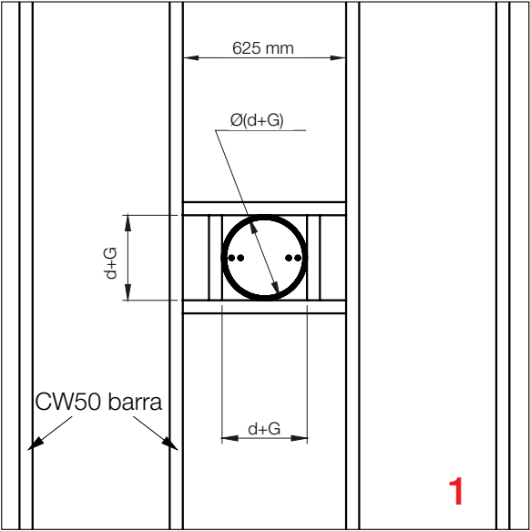
E-FDC-MF2 Serranda tagliafuoco ( \varnothing d < 625 mm) installazione in parete di vani (90 mm) con borchie metalliche
