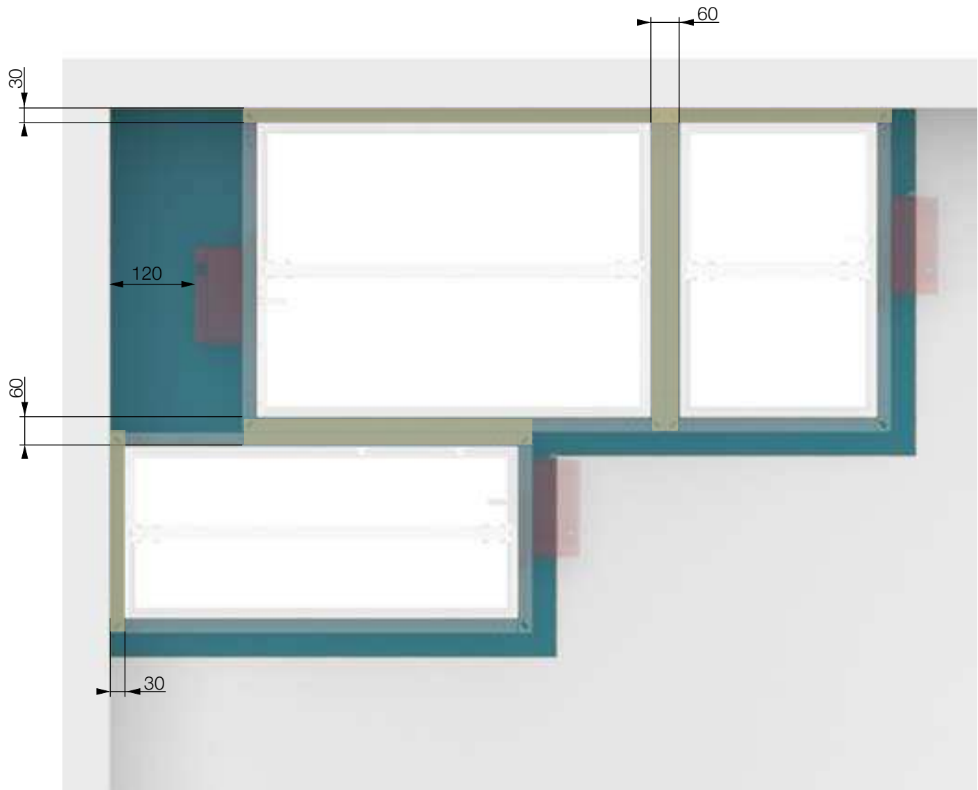
* Distanze minime tra le serrande o parete/soffitto.
