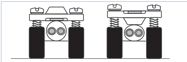
Montage des Netzkabels unter der Zugentlastung
